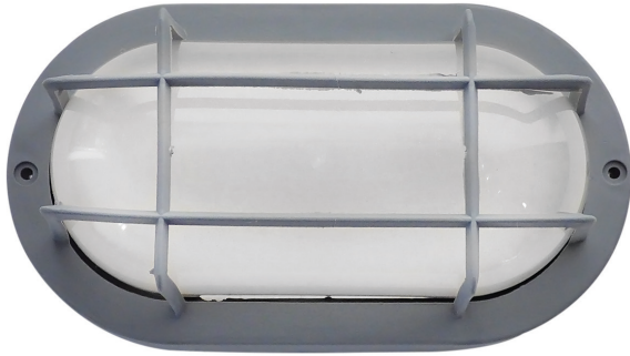
SLP-400 GREY 13-0011 H11 x 20,5 x 10,5 cm E/27 max 11w LED ή EL IP 23
